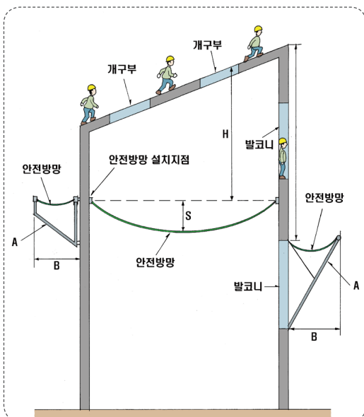
안전방망의 설치방법
