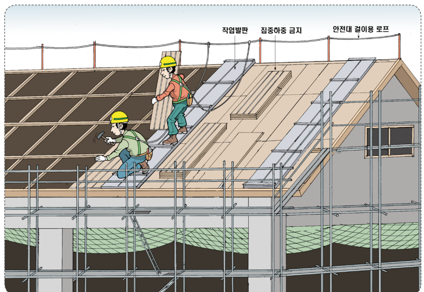
경사진 지붕 안전시설 설치(예)
