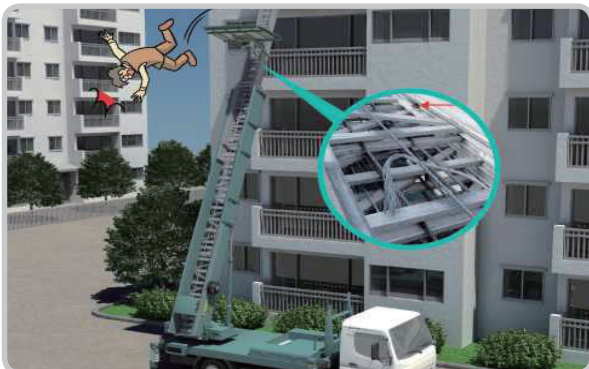
▲ 보조 와이어로프 풀림에 의한 충격으로 떨어짐
