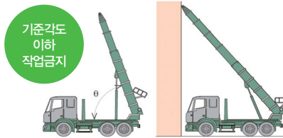
기준각도 이하 작업금지 제작사 설계기준에서 정하는 각도 이하 작업금지
