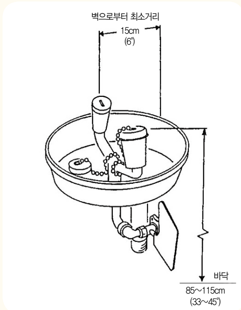
세안설비의 예
