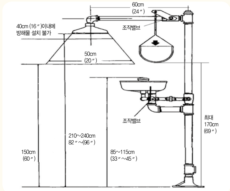
샤워기와 세안설비 결합 설치 예
