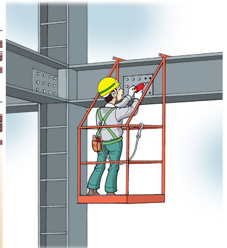
〈철골작업 달대비계 사용 예〉
