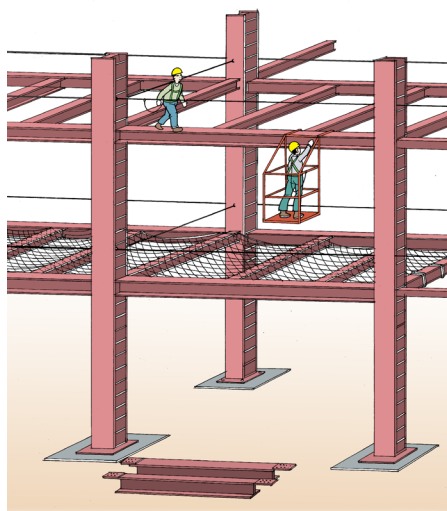
〈철골작업 시 안전시설 설치 예〉
