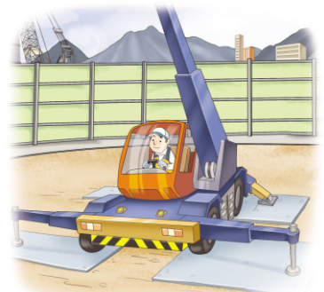
연약지반 깔판설치
