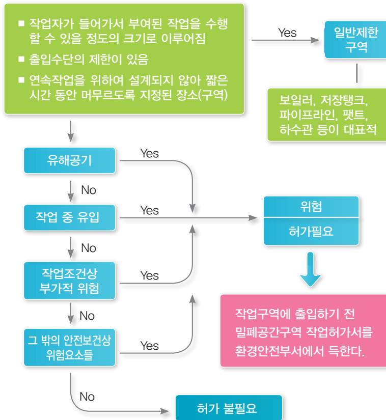
[ 밀폐공간 작업 허가 흐름도 ]
