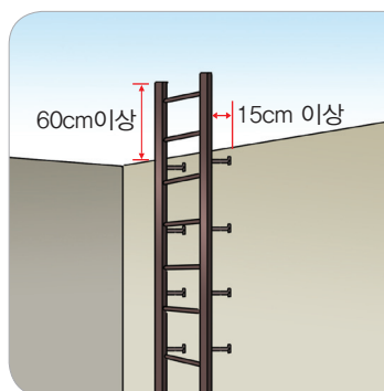
올바른 사다리 설치
