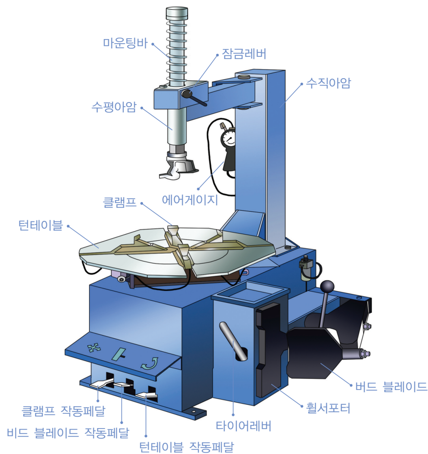
타이어 탈착기 구조
