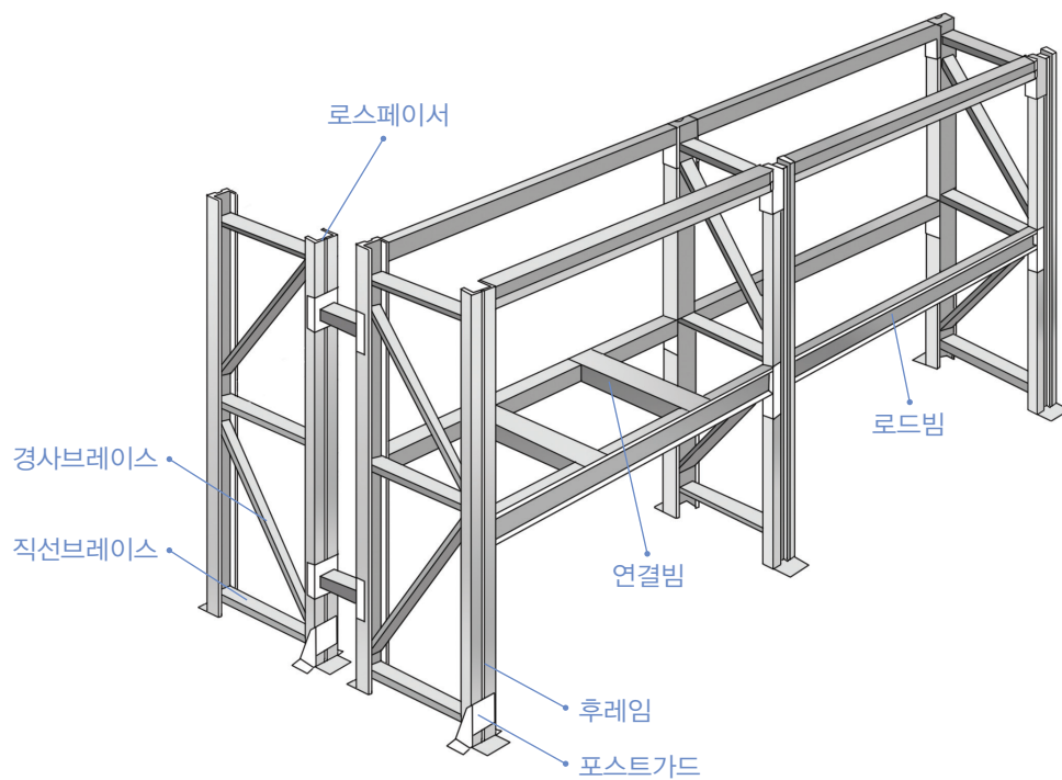
파렛트 랙 구조
